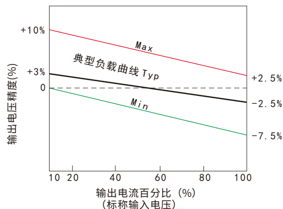
误差包络曲线图 5Vdc输出
