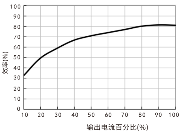
效率Vs输出负载(Vin=24V) F2405D-1WR3
