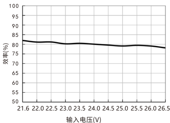
效率Vs输入电压(满载) F2405D-1WR3
