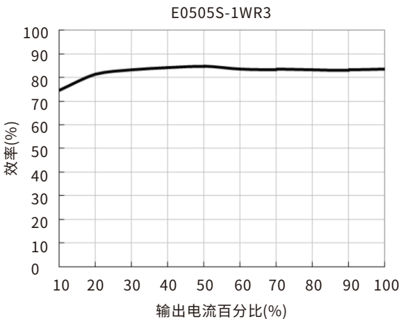
效率Vs输出负载(Vin=5V)
