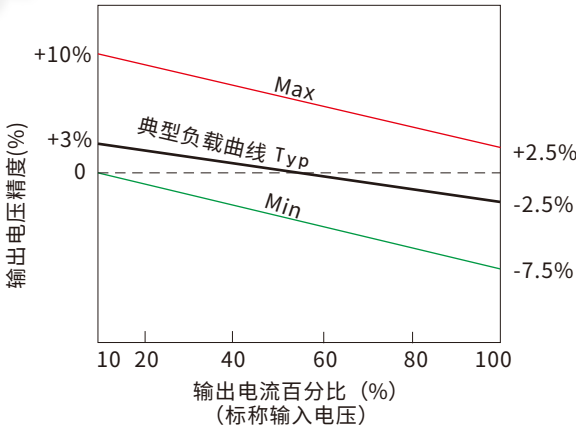
误差包络曲线图 5Vdc输出
